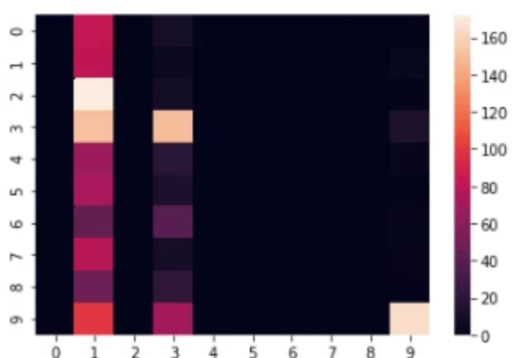
図 19 発動機能推定結果の混同行列のヒートマップ (線形 SVM) 0:Kindle, 1:AmazonMusic, 2:ビデオ通話, 3:質問, 4:News, 5:AmazonPrimeVideo, 6:レストラン検索, 7:Spotify, 8:TuneIn, 9:音声通話
