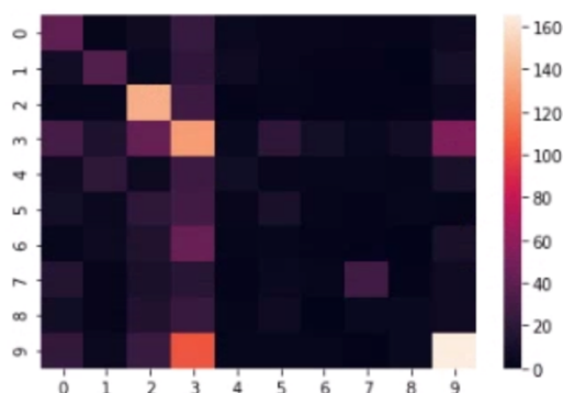
図 18 発動機能推定結果の混同行列のヒートマップ (K 近傍) 0:Kindle, 1:AmazonMusic, 2:ビデオ通話, 3:質問, 4:News, 5:AmazonPrimeVideo, 6:レストラン検索, 7:Spotify, 8:TuneIn, 9:音声通話
