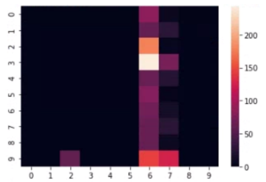
図 16 発動機能推定結果の混同行列のヒートマップ (SGD)
