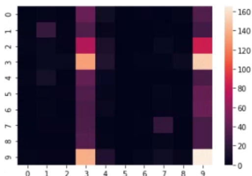
図 20 発動機能推定結果の混同行列のヒートマップ (カーネル近似) 0:Kindle, 1:AmazonMusic, 2:ビデオ通話, 3:質問, 4:News, 5:AmazonPrimeVideo, 6:レストラン検索, 7:Spotify, 8:TuneIn, 9:音声通話
