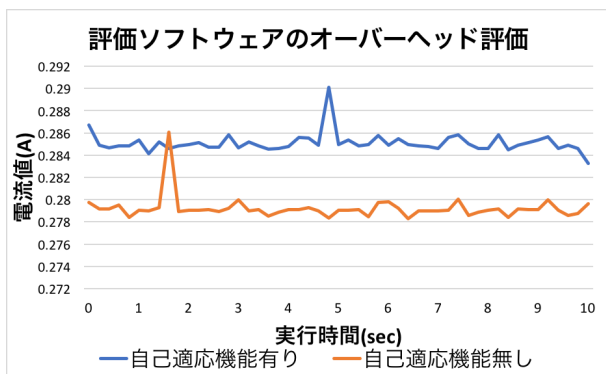
図 10 評価ソフトウェアのオーバーヘッド評価
