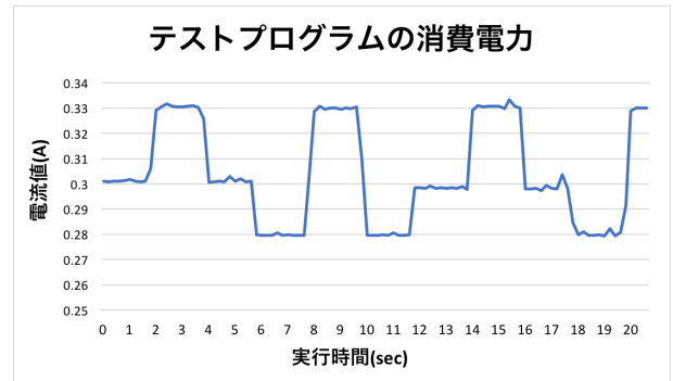
図 8 テストプログラムの消費電力 Fig. 8 Power consumption of the test program
