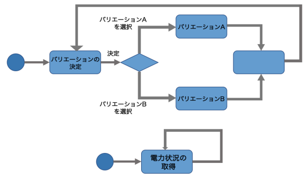
図 5 電力状況の取得とバリエーションの変更 Fig. 5 Power situation acquisition and variation change
