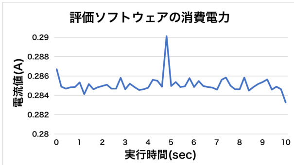
図 7 評価ソフトウェアの消費電力 Fig. 7 Power consumption of the evaluation software
