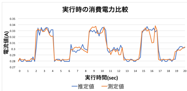
図 9 実行時の実測値と推定値の比較
