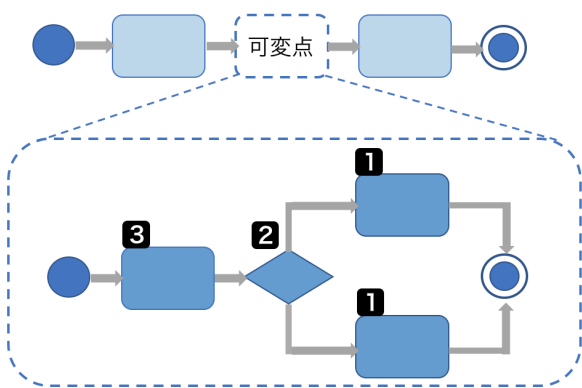
図 2 振る舞いのモデルのメタモデル
