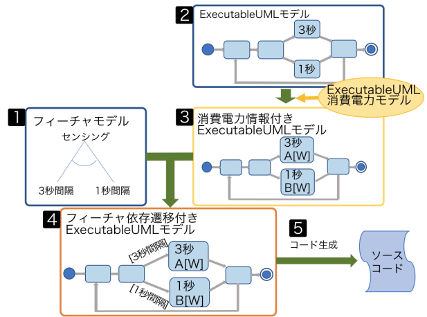
図 1 開発手法の全体像
