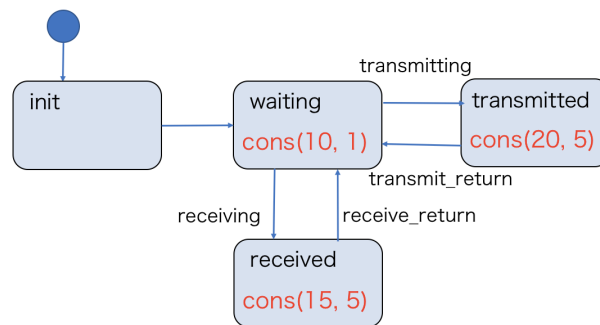
図 3 モデルベース消費エネルギー解析手法の全体像
