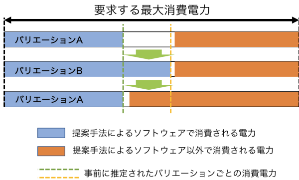
図 4 実行時の振る舞い Fig. 4 Runtime behavior
